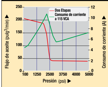
ZW3 Flujo de aceite y corriente en función de la presión hidráulica
