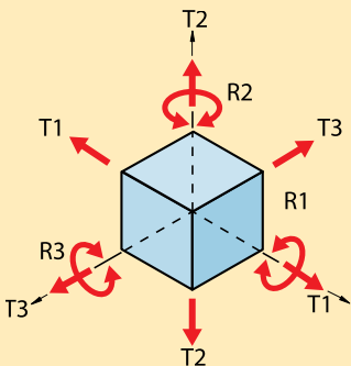
Figura 2 Cuerpo tridimensional
