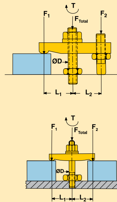
Figura 3 Configuración típica de sujeción mecánica
