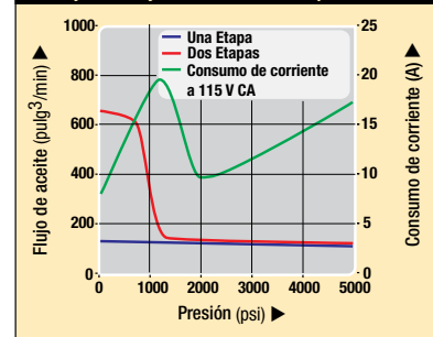
ZW5 Flujo de aceite y corriente en función de la presión hidráulica
